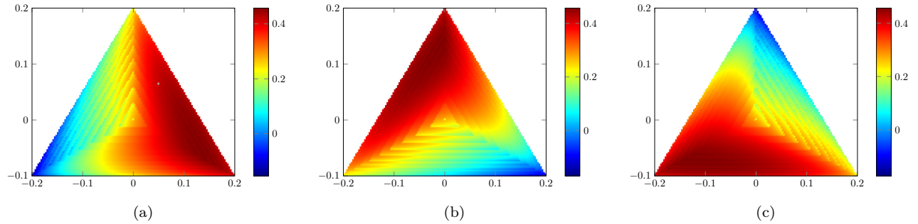
Figura 3: Valor de la carrera de los actuadores en función de la posición (x, y) del efector, (a) para el actuador b_1 . (b) para el actuador b_2 . (c) para el actuador b_3 .
